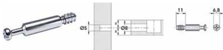
Stift kastverbinding type 21402090ZN
