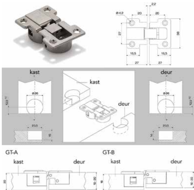
Valdeurscharnier type Ankor
