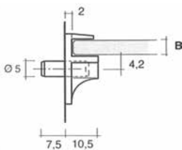
Schapdrager type 34
