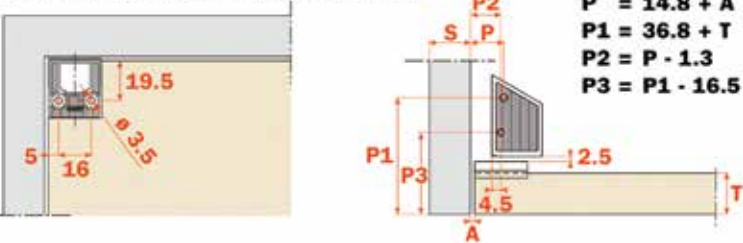
Met Push duwspingslot DP4SNG (032740)
