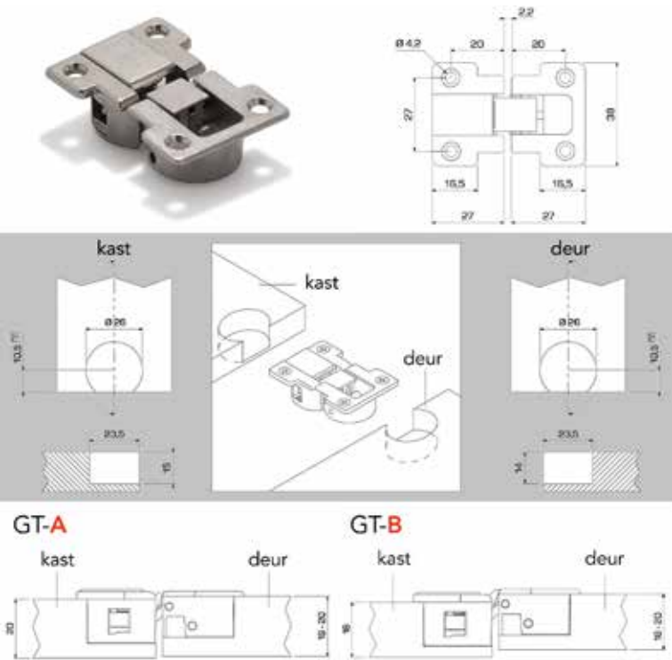
Valdeurscharnier type Ankor voor valdeurbeslag
