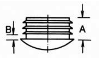
Stoeldop type SRL
