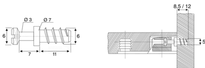
Stift voor Modulfix kastverbindingen
