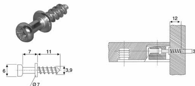
Stift voor Modulfix kastverbindingen
