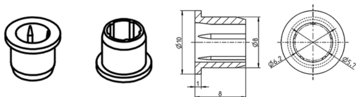
Mof voor houders voor de presentatie van keukenfronten
