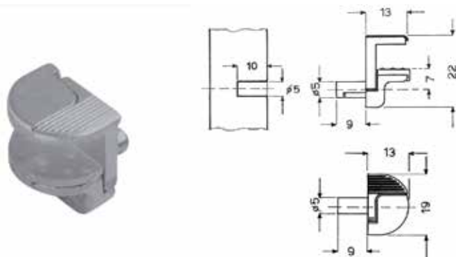
Schapdrager type Alfa
