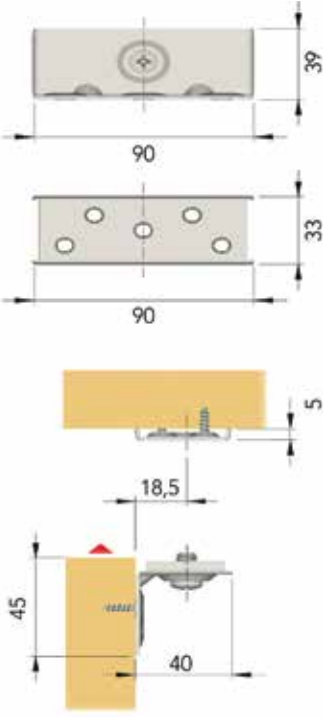
Bedbeslag type 03.145.36
