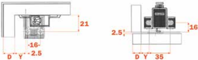
Met Push duwspingslot DP4SNG (032740)
