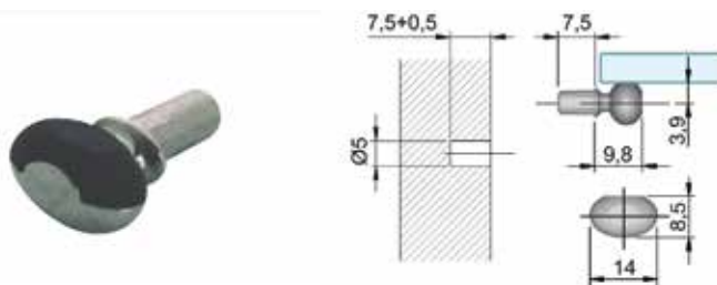
Schapdrager type 3011 van 4 stuks
