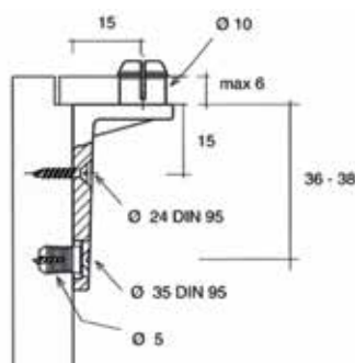
Rugwandklem type 57.0570
