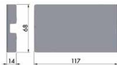
Afdekkap voor valdeurbeslag type Kiaro Easy
